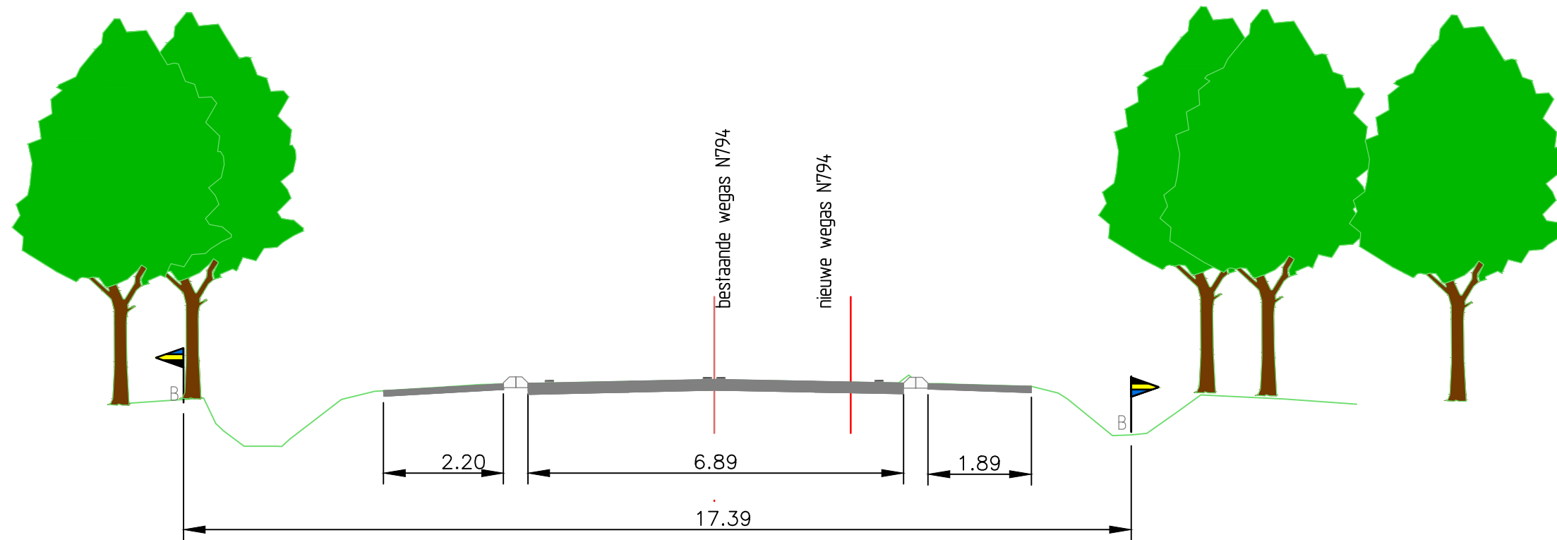
principe dwarsprofiel 3-3 traject 3 locatie km.15.20
