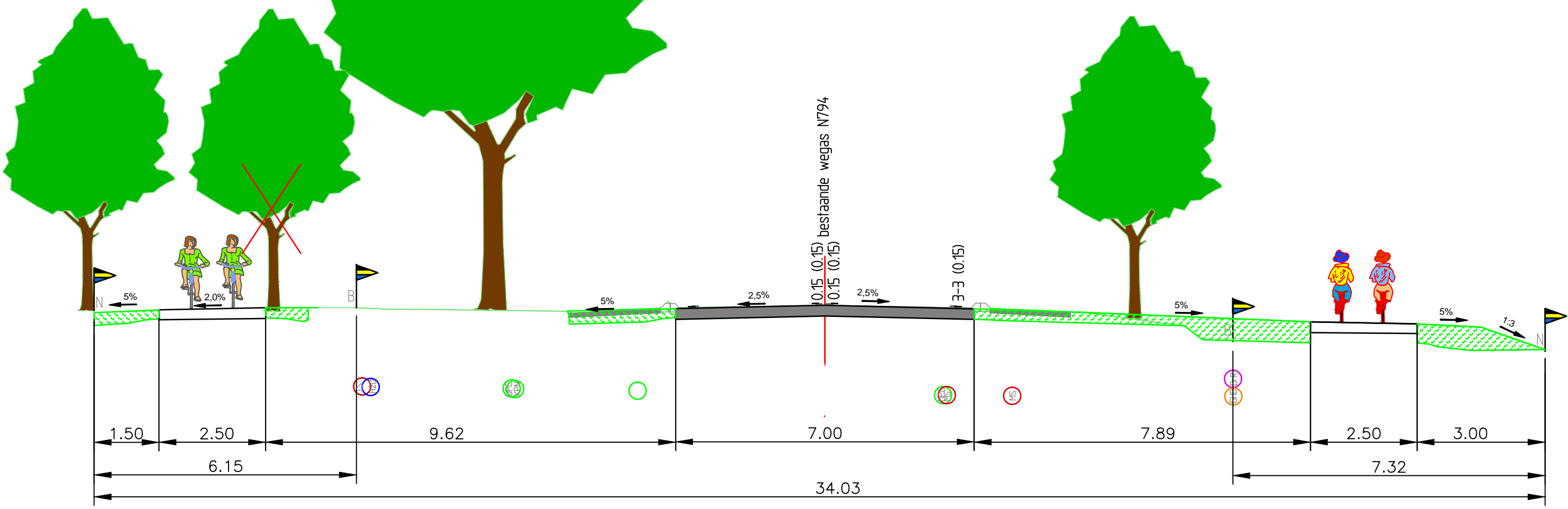
bestaand dwarsprofiel 5-5 traject 3 locatie km.15.70
