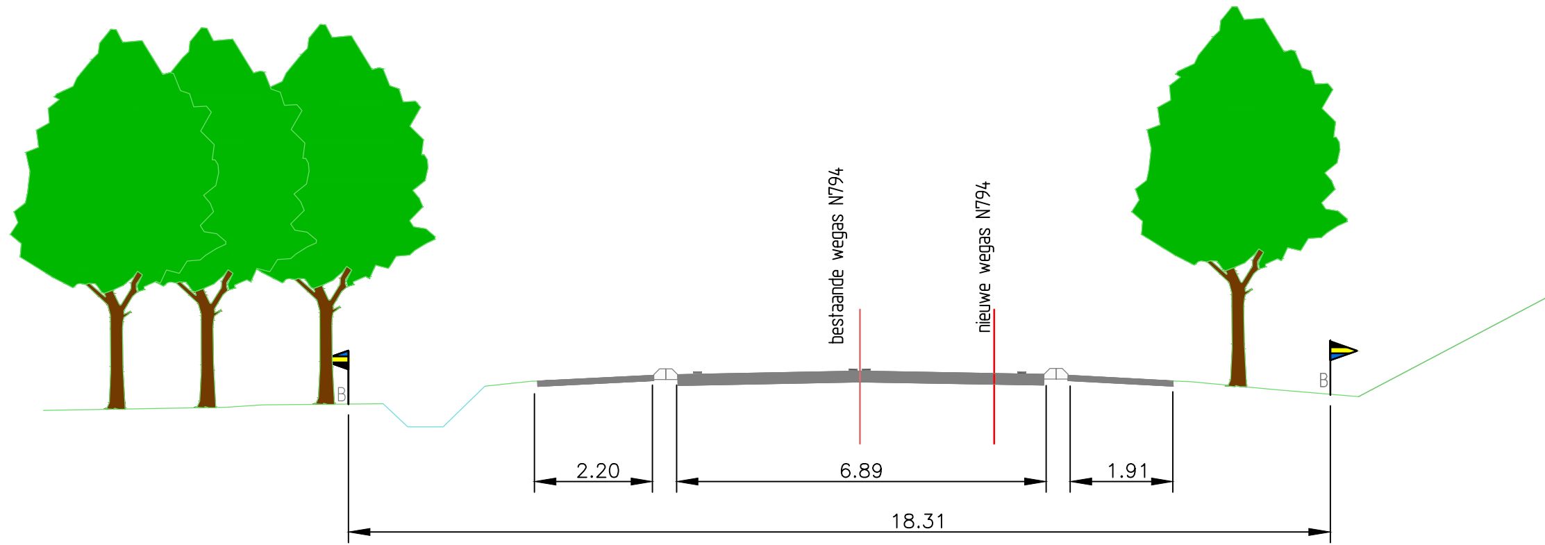
bestaand dwarsprofiel 4-4 traject 3 locatie km.15.30
