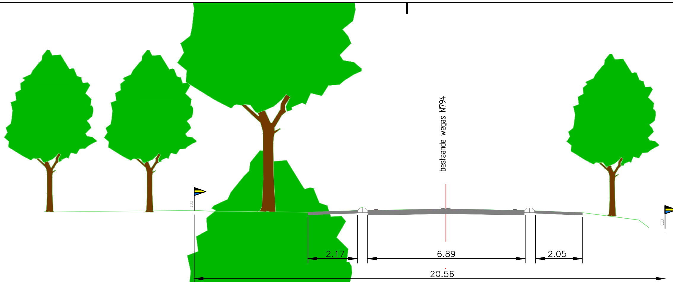
bestaand dwarsprofiel 5-5 traject 3 locatie km.15.70
