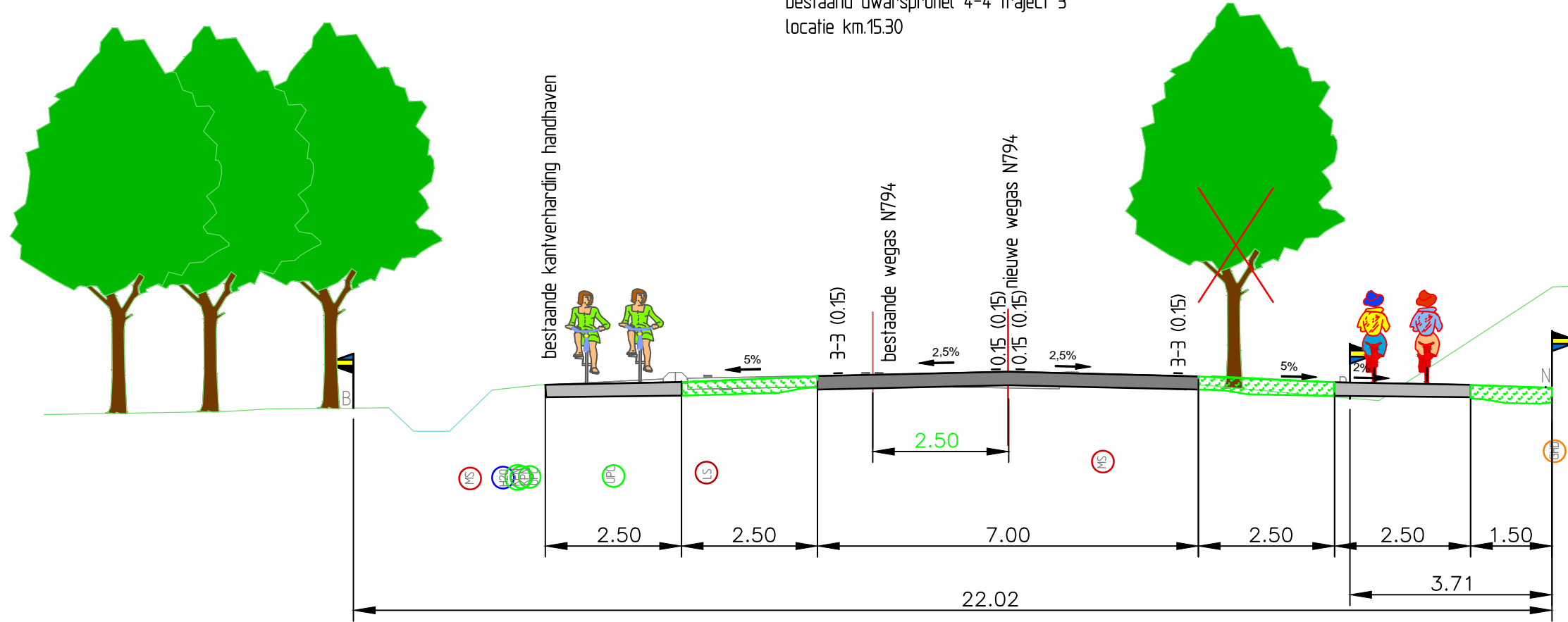
principe dwarsprofiel 4-4 traject 3 locatie km.15.30
