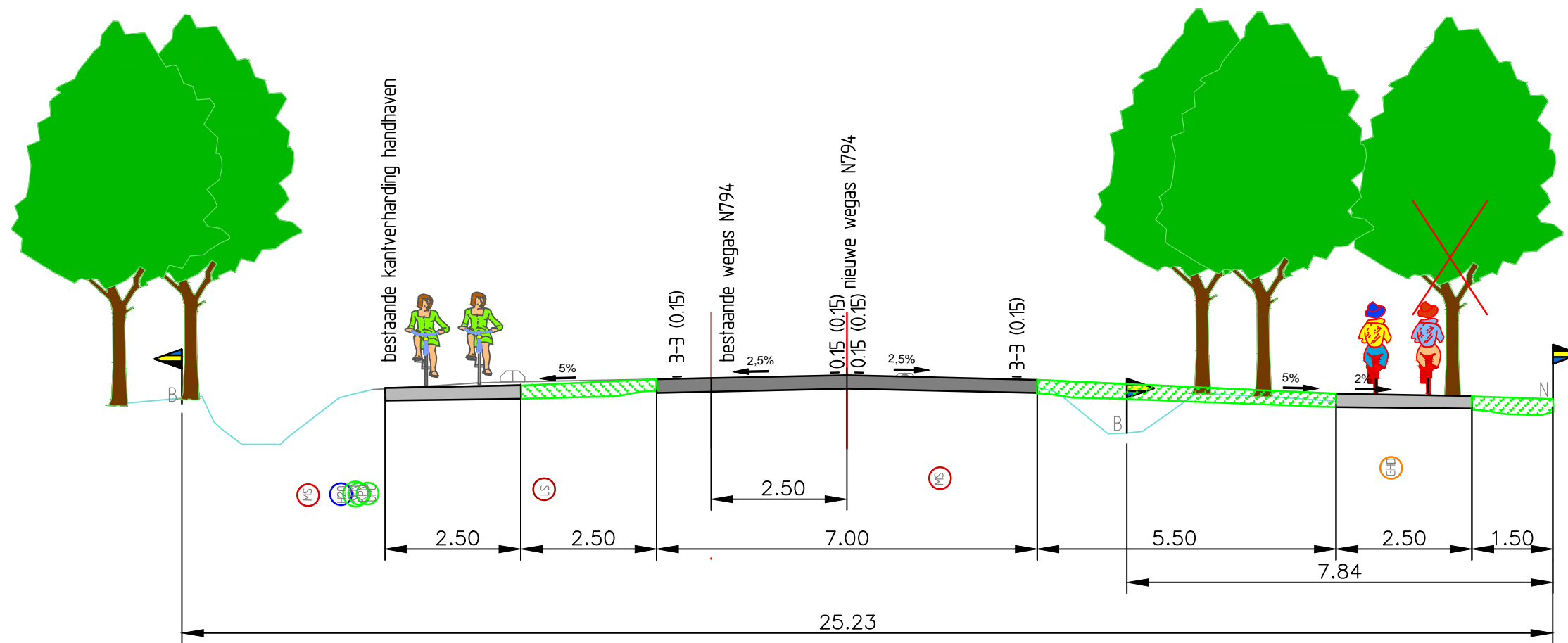
principe dwarsprofiel 3-3 traject 3 locatie km.15.20
