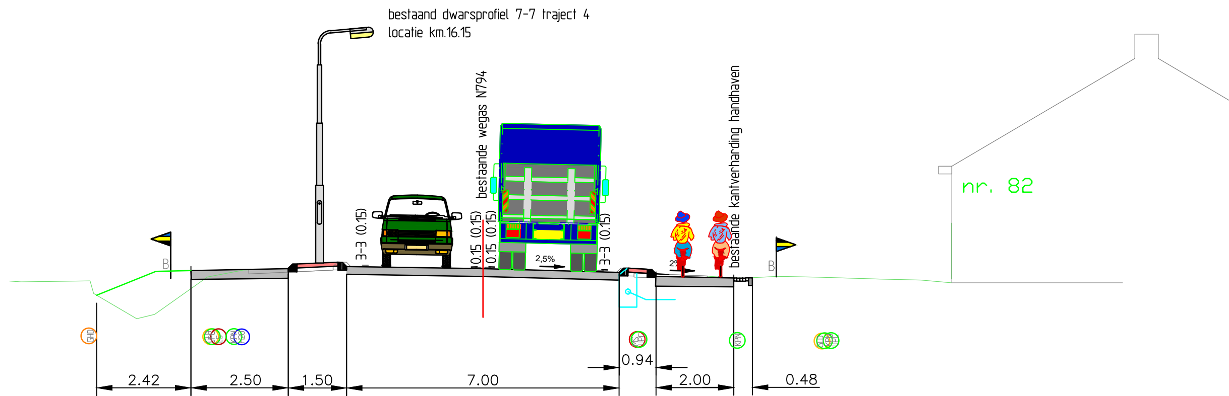
bestaand dwarsprofiel traject 4 locatie km.16.15
